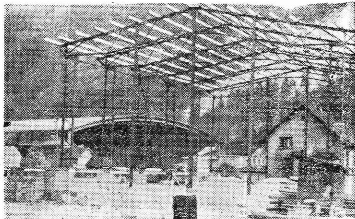
Na severni strani ceste proti strelišču delavci podjetja Kovinoservis Jesenice, postavljajo halo za podjetje Športmetal Jesenice. V njej bodo krivili in pripravljali debelejša betonska železa za gradbeno podjetje.
