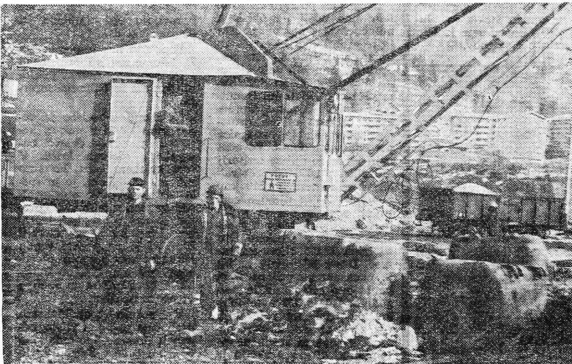
»Svinje«, ki jih potegnejo izpod peči v jeklarni, razbijajo in pri tem ločijo od žindre še uporabno železo, ki ga zrežejo in zopet pošljejo v talilnice. Na sliki sodelavci pri tirnem dvigalu »slon«, na prostoru za čiščenje »svinj«
