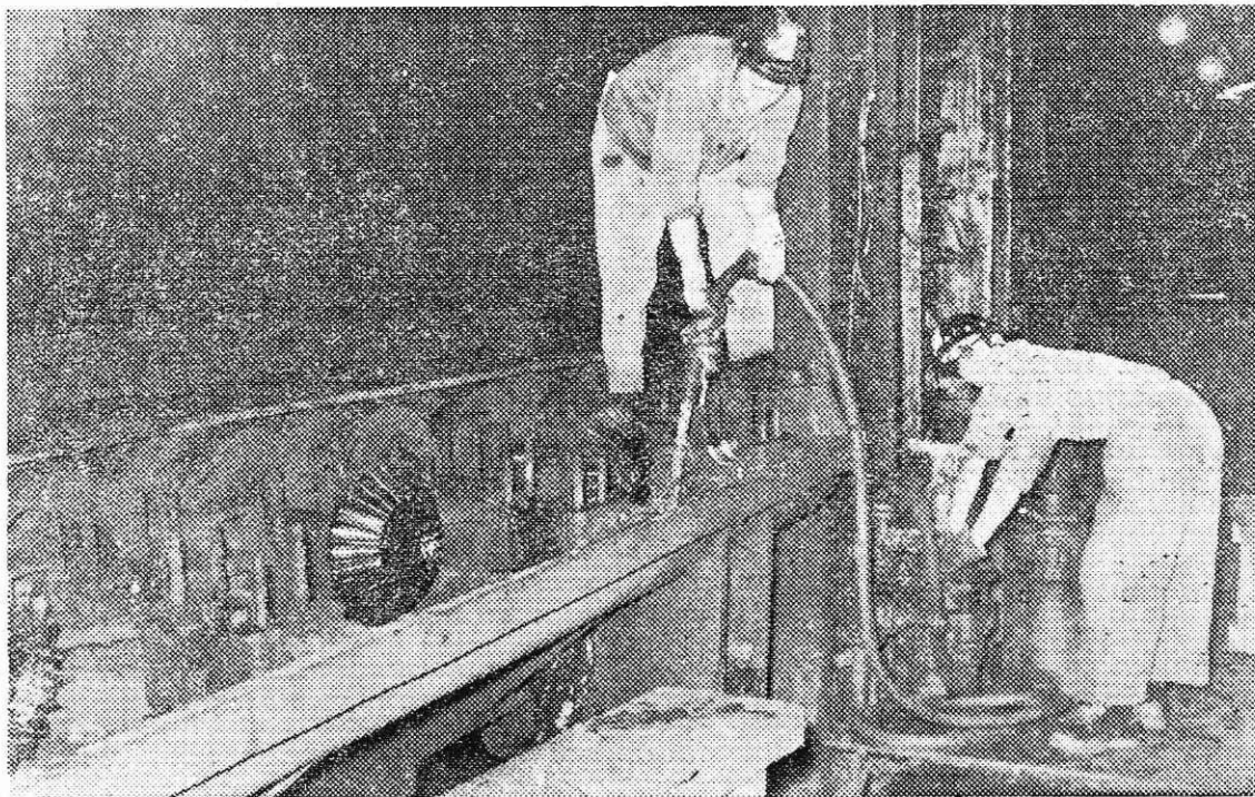
Generalni remont valjarne 2400 je bil opravljen po programu.
