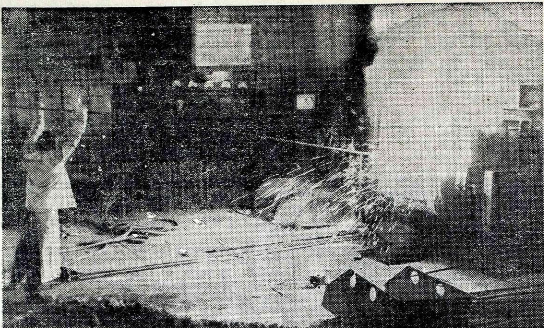
Osemtonska BBC električna peč
