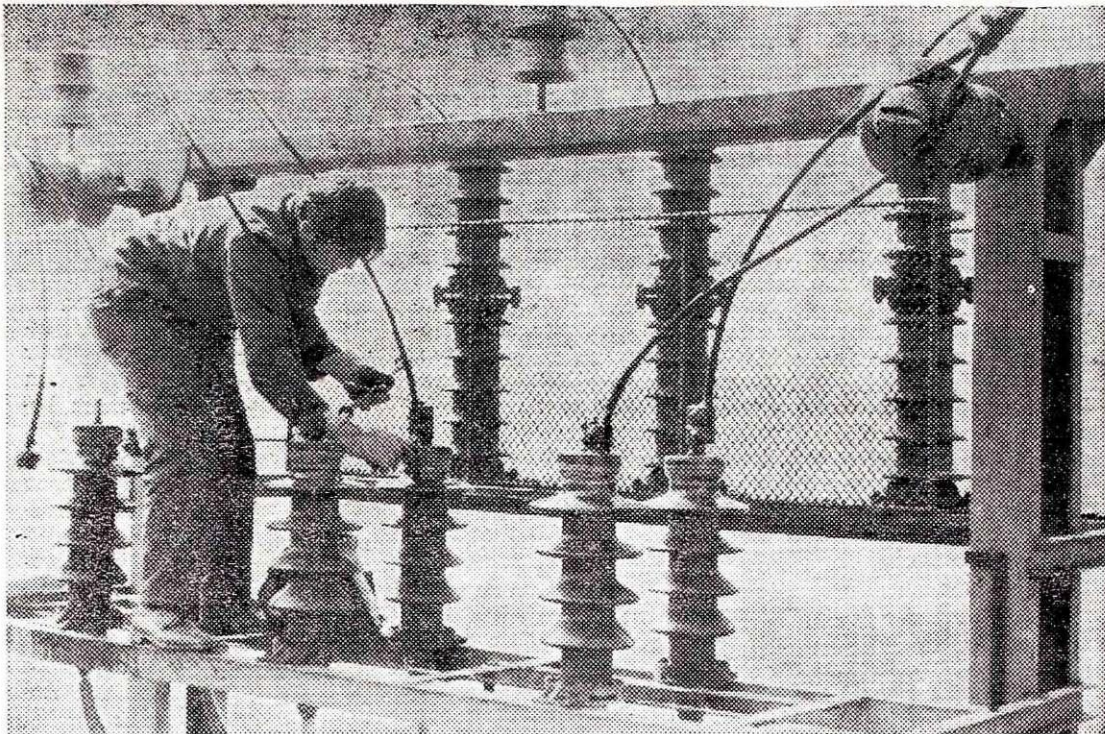
Elektrikar pri popravilu 35 kW glave na portalu dalnovoda Bela
