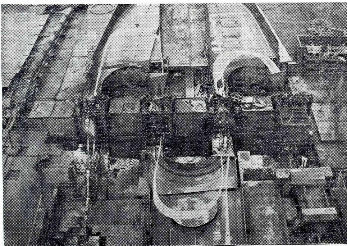
Proga Ø 270 v valjarni žice na Beli
