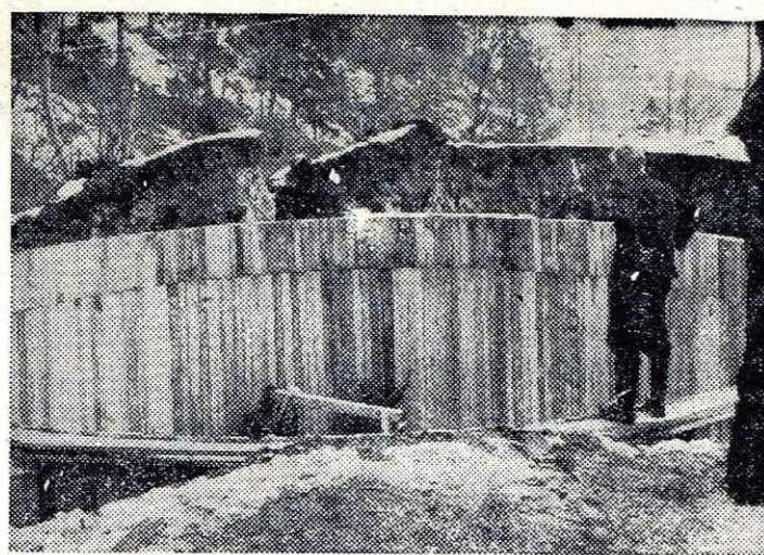
Zajetje vode med gradnjo na Koroški Beli
