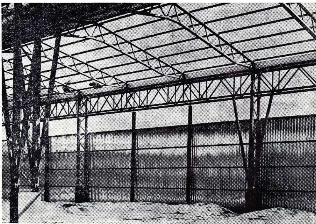
Konstrukcija iz hladno oblikovanih profilov skladišča UNIVERZAL
