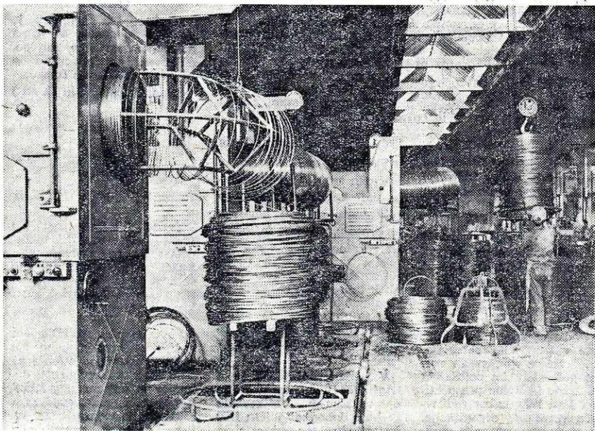
Žičarski stroji HERBORN — šeste in osme stopnje
