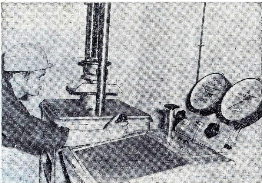
Stiskalnice za določanje mehanske in upogibne trdnosti (firme Tonindustrie, Berlin) uporabljamo pri preiskavah vseh vrst ognjeodpornih materialov. Vzorec v obliki kocke (50 x 50 mm) ali valja (50 x 40 mm) vstavimo v stiskalnico in počasi obremenjujemo vzorec tako, da dvigamo pritisk. Pod določeno obremenitvijo se vzorec zdrobi. Iz površine vzorca in odčitane obremenitve na instrumentu izračunamo tlačno trdnost. S to napravo lahko določujemo maksimalne trdnosti do 800 kp/cm 2 .
