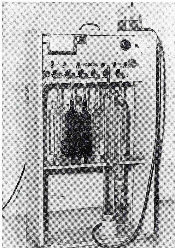
Orsat aparat za določevanje industrijskih plinov.
