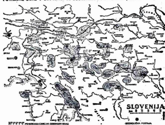
Slika 23: Cone potresov
