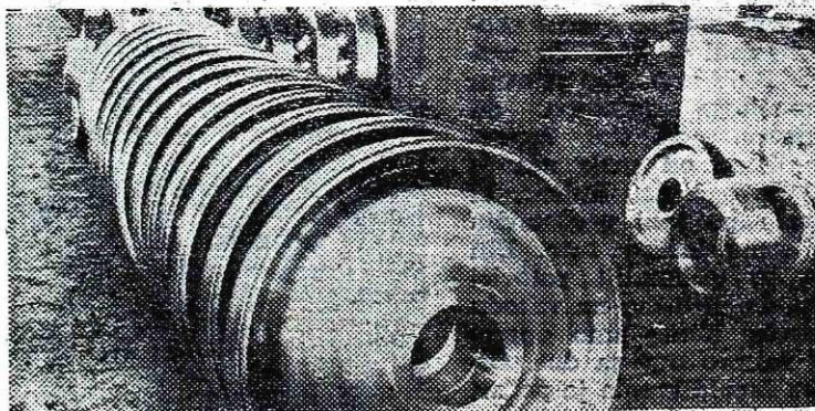
Kolesa za železniške vozove — izdelek železarne Ravne
