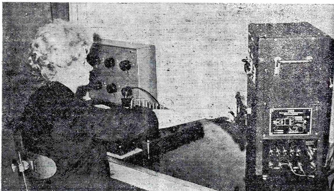
RO — aparat za merjenje magnetnih lastnosti elektropločevine
