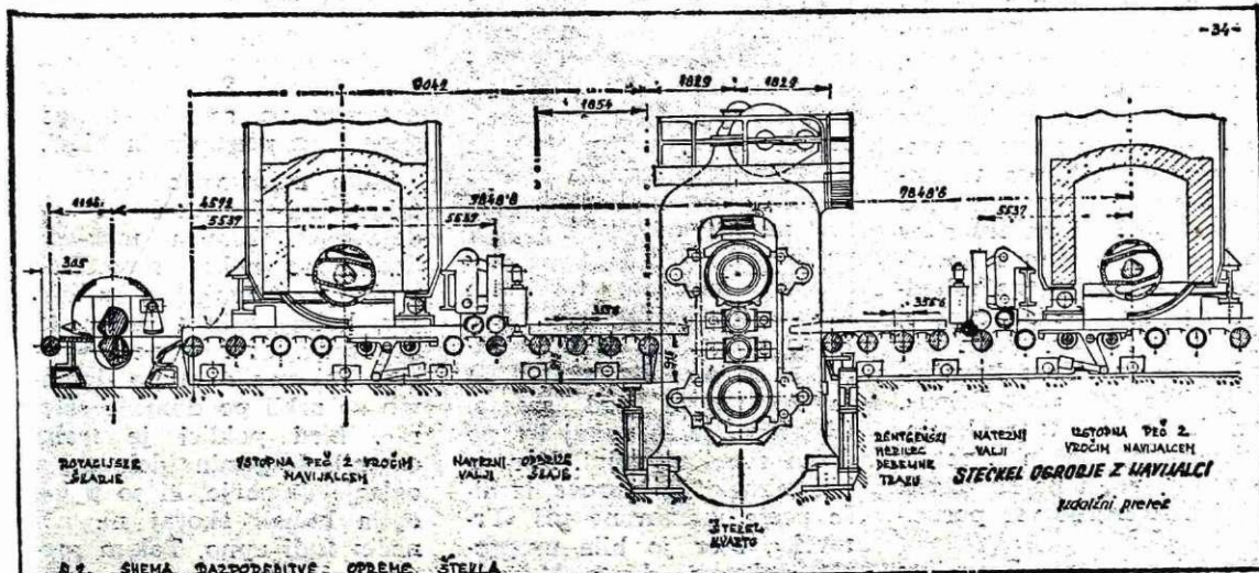
Shema razporeditve opreme štekla
