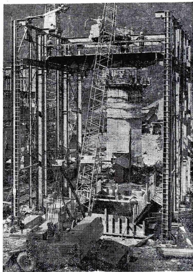
Montaža mačka na enem izmed objektov aglomeracije
