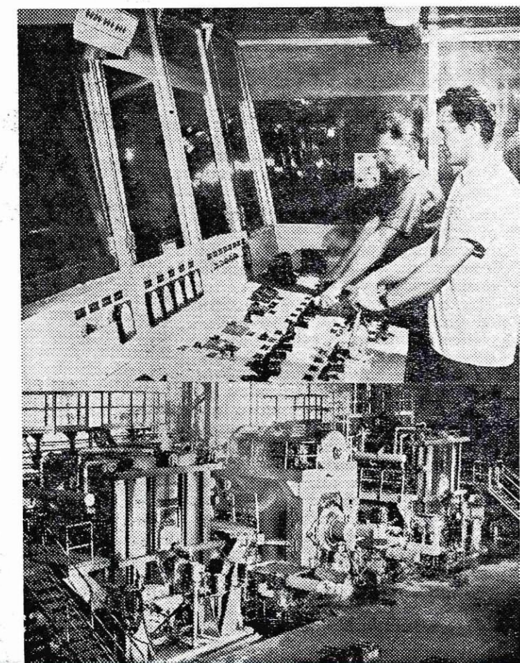
Tehnološki proces valjanja trakov se upravlja iz komandne kabine (zgoraj), spodaj valjarna trakov ŠTEKEL.
