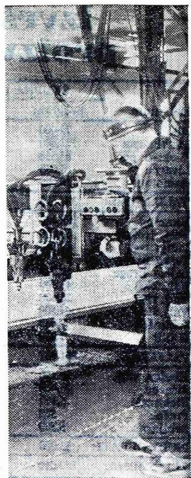
Avtogensko rezanje debele pločevine
