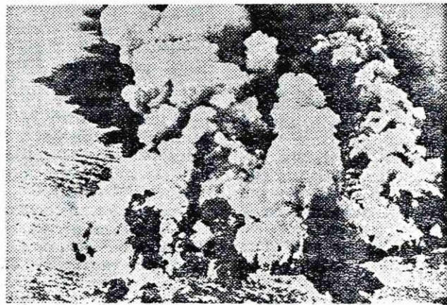
Slika 8. Izbruh podmorskega vulkana na Pacifiku
