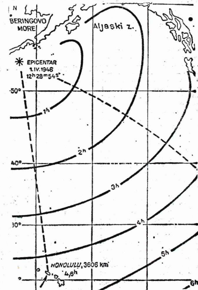
Slika 9. Širjenje potresnih valov »tsunami« od Aleutskega grebena do otočja Honolulu. Dobro so vidni koncentrični krogi širjenja »tsunami«
