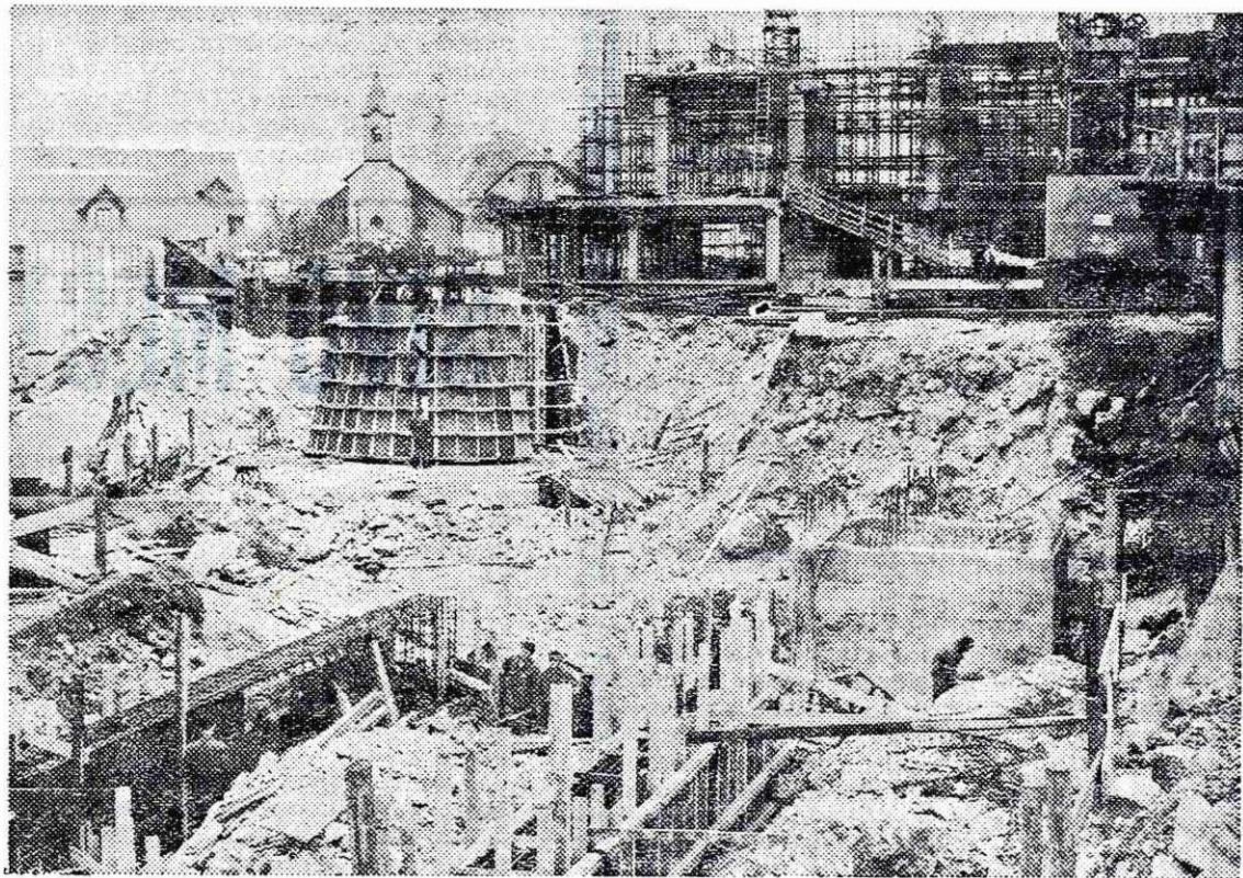
Začetek gradnje novega dimnika na gradbišču aglomeracije
