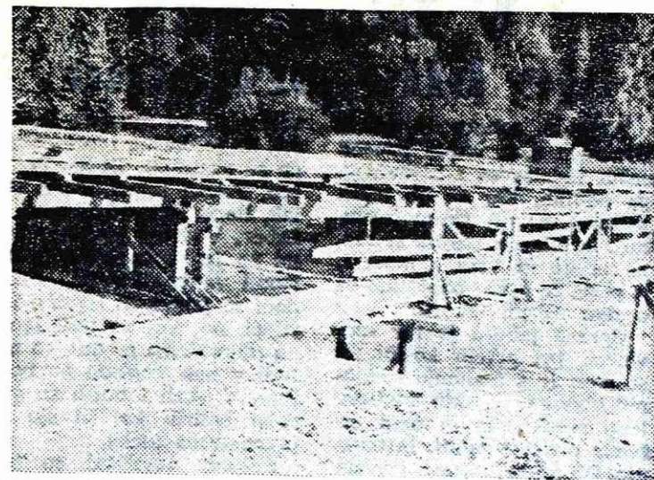
PRI MOJSTRANI GRADE NOV MOST ČEZ SAVO DOLINKO — 1966. leta so poplave v jeseni odnesle most čez Savo Dolinko pod Mojstrano. Delavci SGP Sava so lani pričeli graditi novega, ki bo nared do jeseni. Za Mojstrano bo to vsekakor ugodno, ker bo bližje do vasi, pozimi pa do novega smučišča in žičnice.
