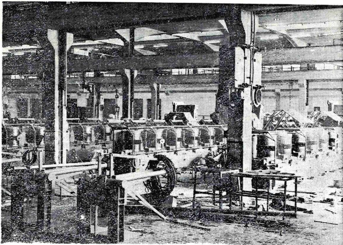
Tudi oba šeststopenjska žičarska stroja sta pridobitev žičarne
