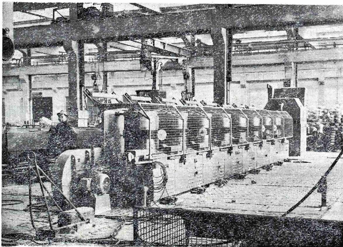
V žičarni so dobili nov osemstopenjski žičarski stroj
