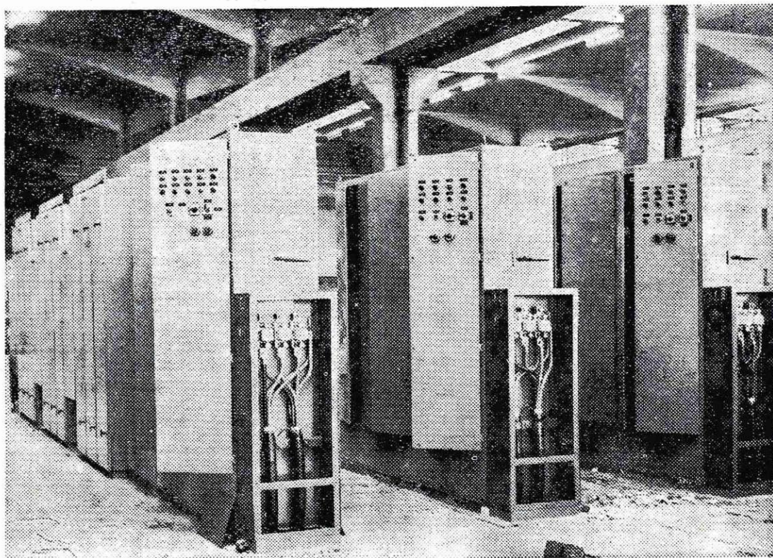
Del novih naprav pri novih žičarskih strojih v žičarni
