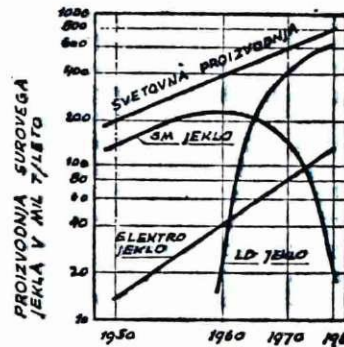
RAZVOJ PROIZVODNJE SUROVEGA JEKLA PO POSAMEZNIH POSTOPKIH
