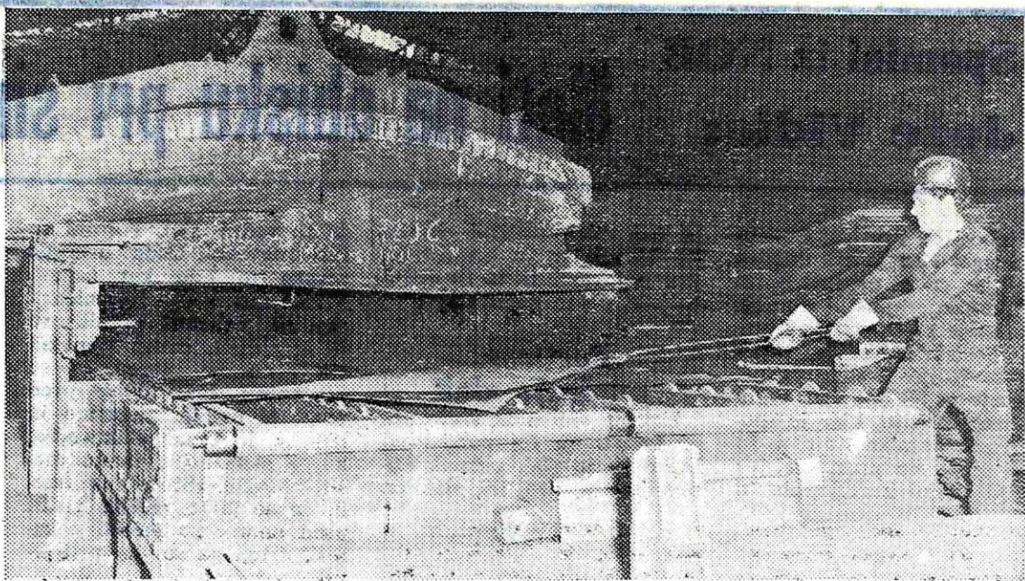
Delavec pri normalizirni peči v valjarni 1300
