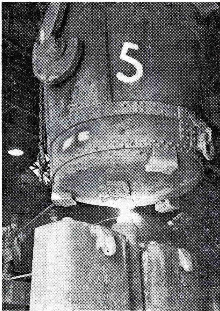
Vlivanje jekla v kokile iz električnih peči
