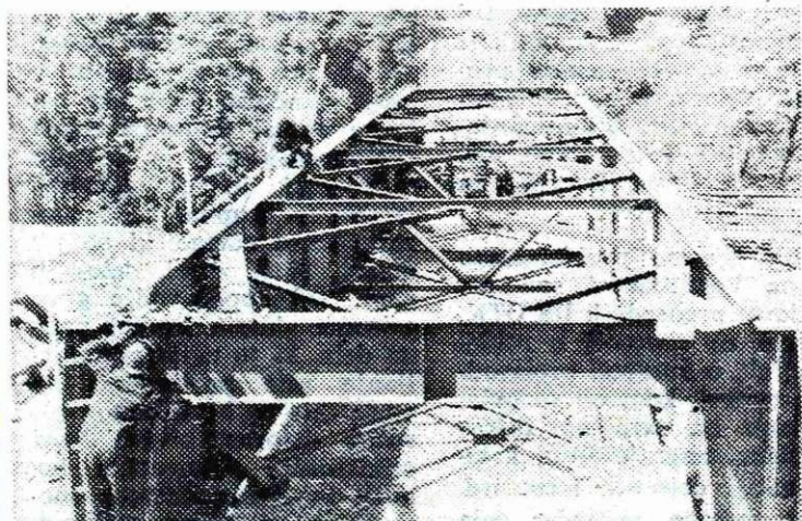
Konstrukcija za nov cestni most v Mostah pri Žirovnici je že na gradbišču
