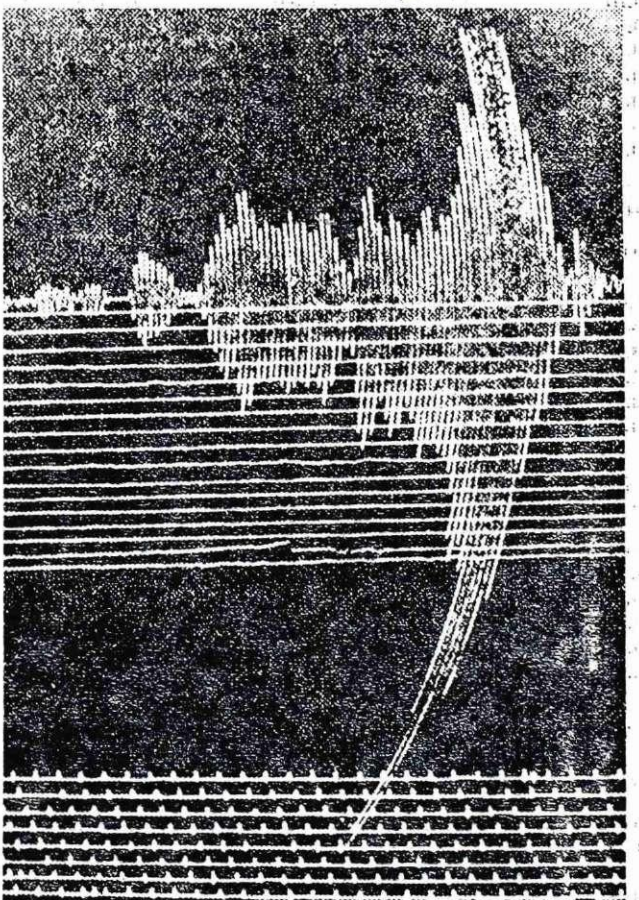
Slika 2 — Seizmogram potresa
