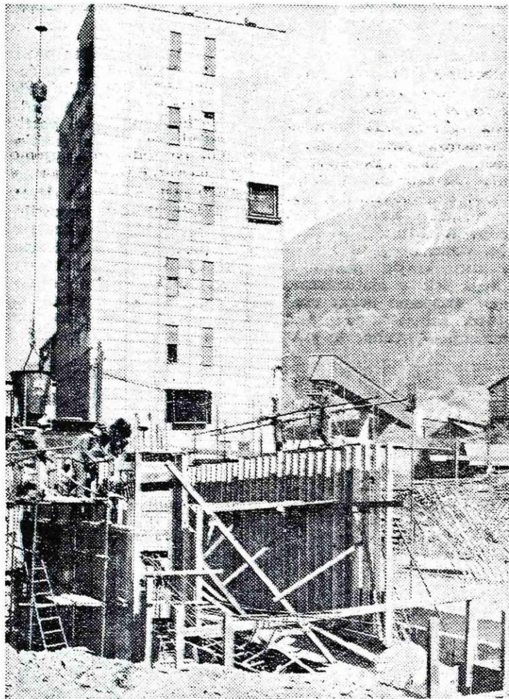
Betoniranje temeljev za objekt »dobilnica rude« v okviru nove aglomeracije
