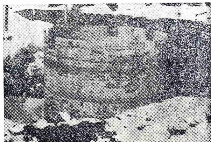
Razbijalnica kokil je bila pod Sava žerjavi. Ker pa je količina kokil od 4 do 8-krat večja, dosedanja razbijalnica ni več kos svojim nalogam, so začeli na nasipu z izgradnjo nove razbijalnice kokil. Na sliki jama, v kateri je velikemu sodu podobna razbijalnica.
