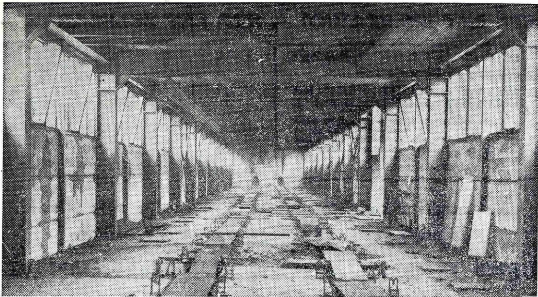
Nova aglomeracija — hala dozirnih silosov v objektu 17
