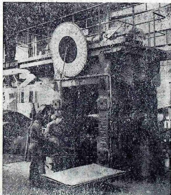
Ogrodje za hladno valjanje pločevine v valjarni 1300
