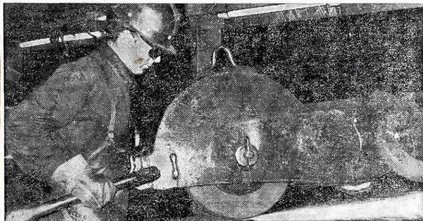
Čiščenje gredic v profilnih valjarnah
