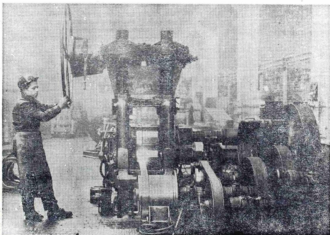
Hladna valjarna — hladno vlečenje trakov
