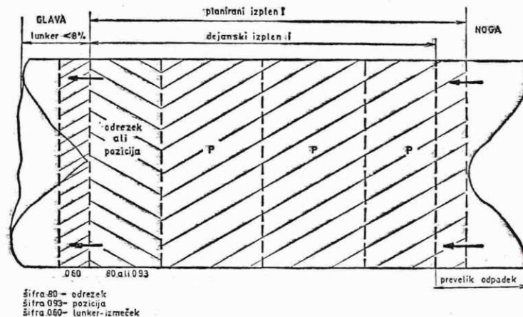
Slika 6 — Vpliv prevelikega odreza na nogi slabov na izplen
