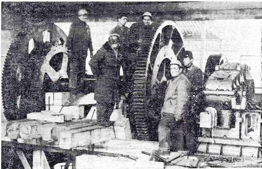
Montaža pogona hladilca sintra (aglomerac.). Šef nadzora za poljsko firmo CENTROZAP Kaptovce in HUTA ZABRZE dipl. inž. Wojnar med delavci
