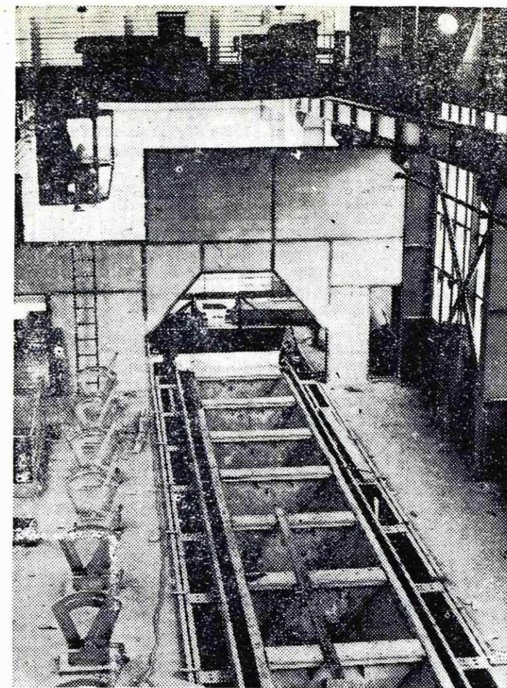
Vakuumske komore sinter stroja (aglomeracija — obj. 22)
