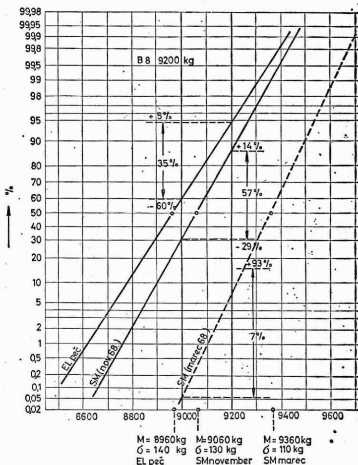
Slika 3 — Statistična analiza tež bram B 8 — 9.200 kg.
