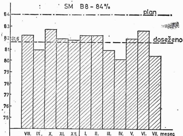
Slika 1 — Izplen pri valjanju bram (B 8) SM jekla za slabe.
