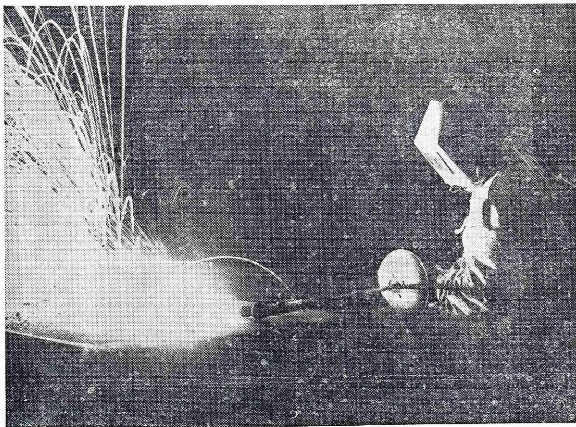
»Flemlanje« slabov v valjarni Bela
