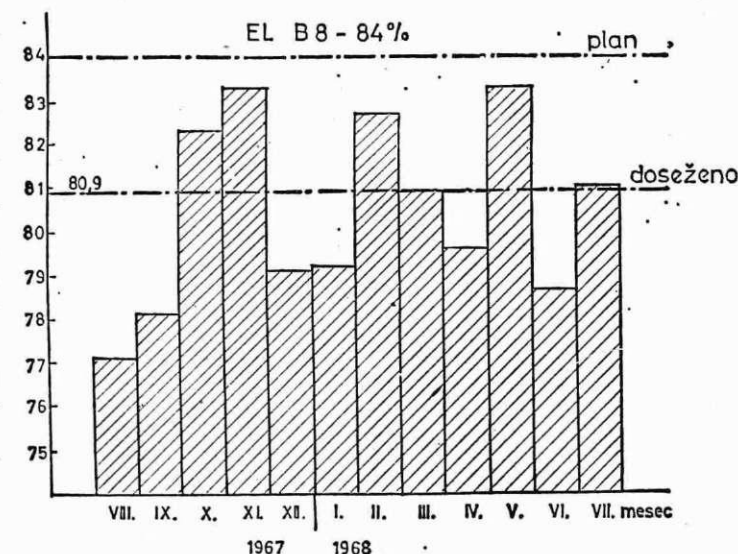
Slika 2 — Izplen pri valjanju bram (B 8) EL jekla za slabe.
