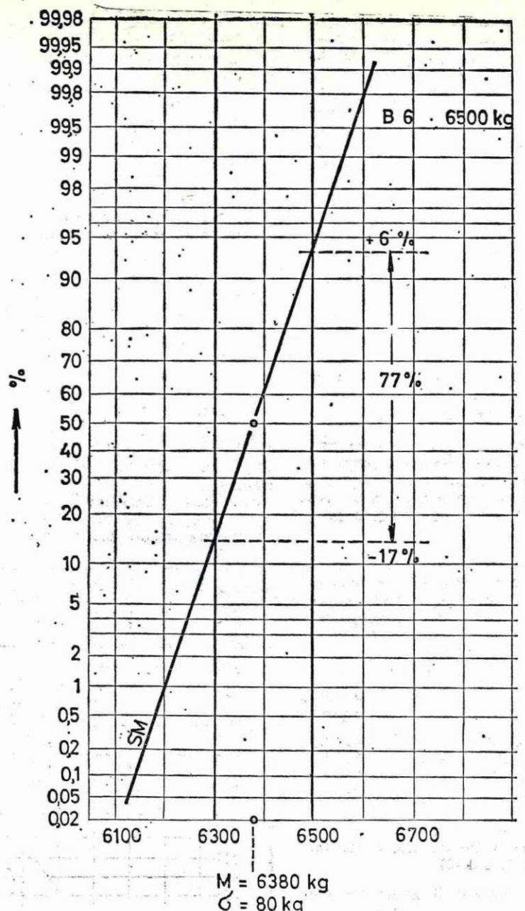
Slika 4 — Statistična analiza vlitih tež bram B 6 — 6.500 kg
