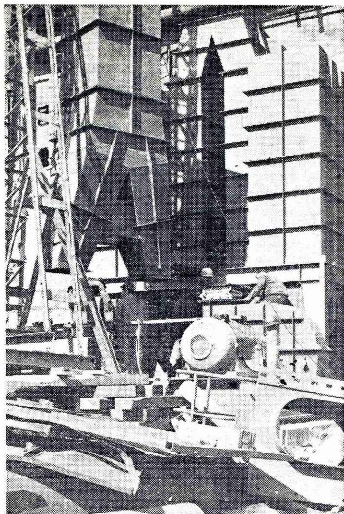
Montaža dimnika za električni peči ASEA in LEKTORMELT
