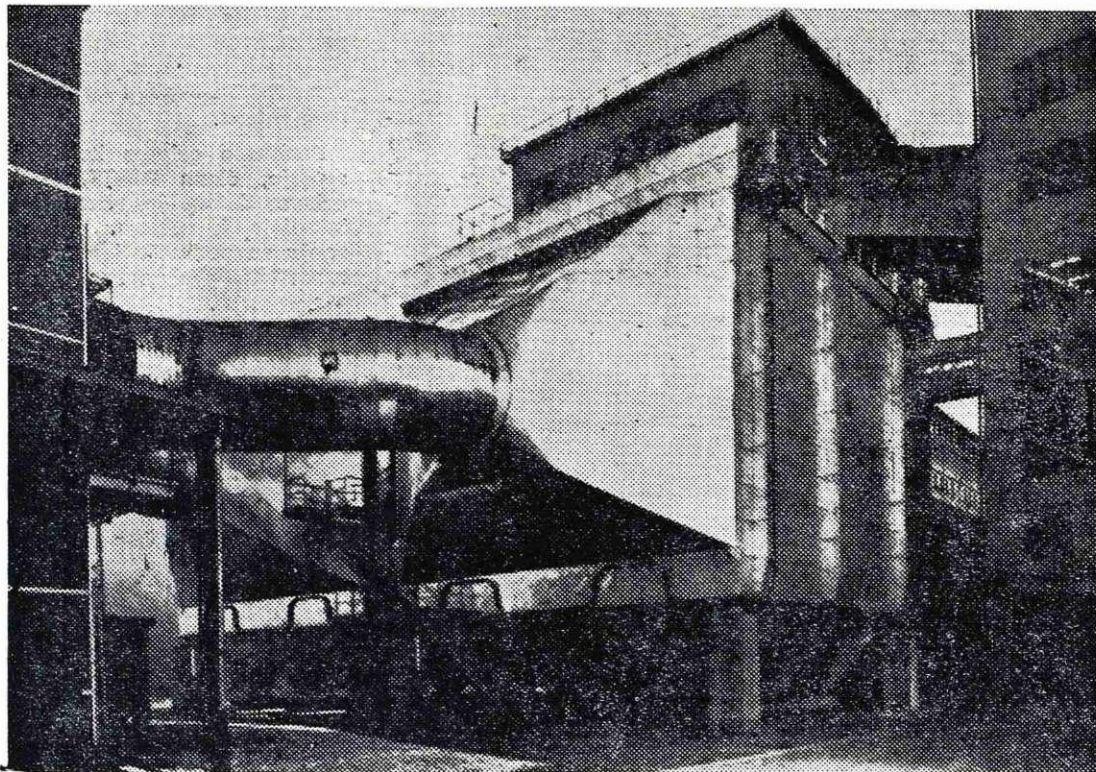
Elektrofilter za oddvajanje dimnih plinov, kakršnega bomo zgradili tudi na Jesenicah
