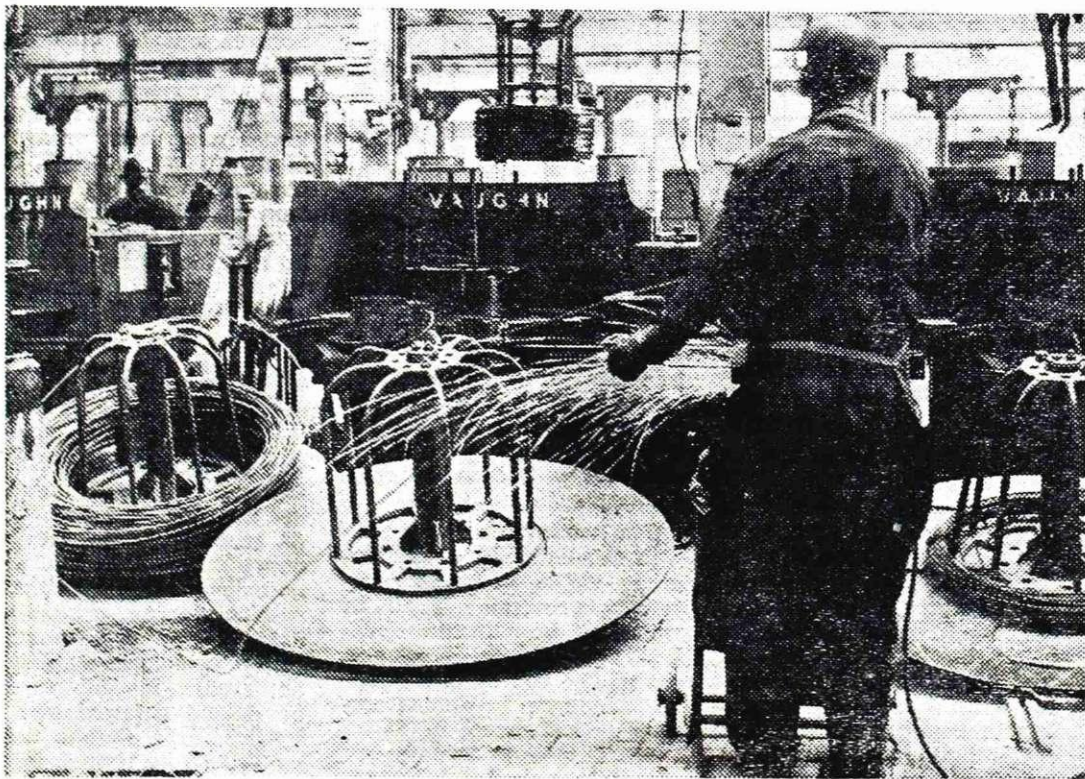
Delo na žičarskem stroju VAUGHN
