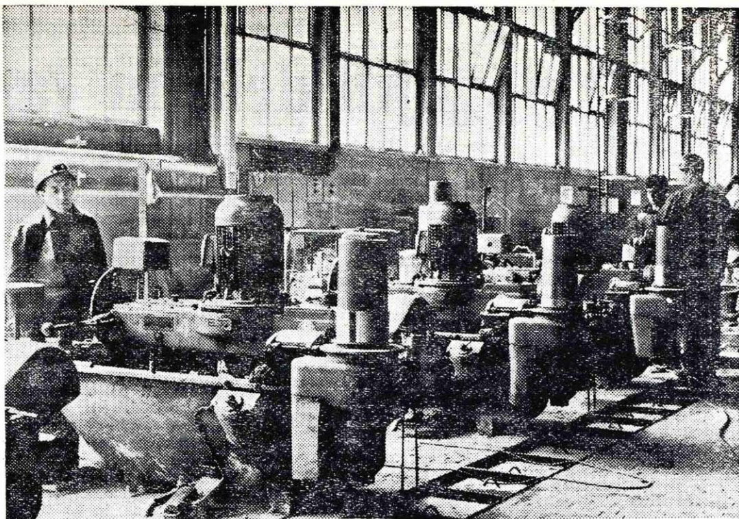
Patentirni stroji za vlečenje žice v patentirnici
