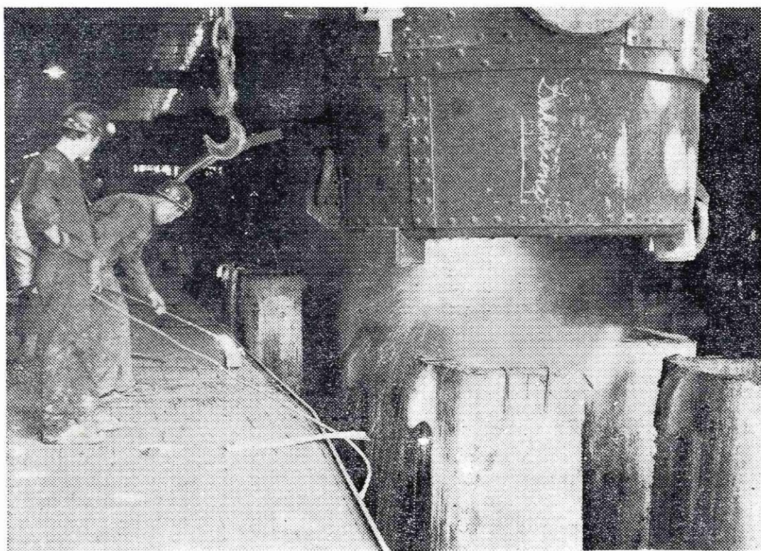
Vlivanje jekla v kokile in zajemanje poskusnega vzorca za laboratorijsko analizo — elektrojeklarna
