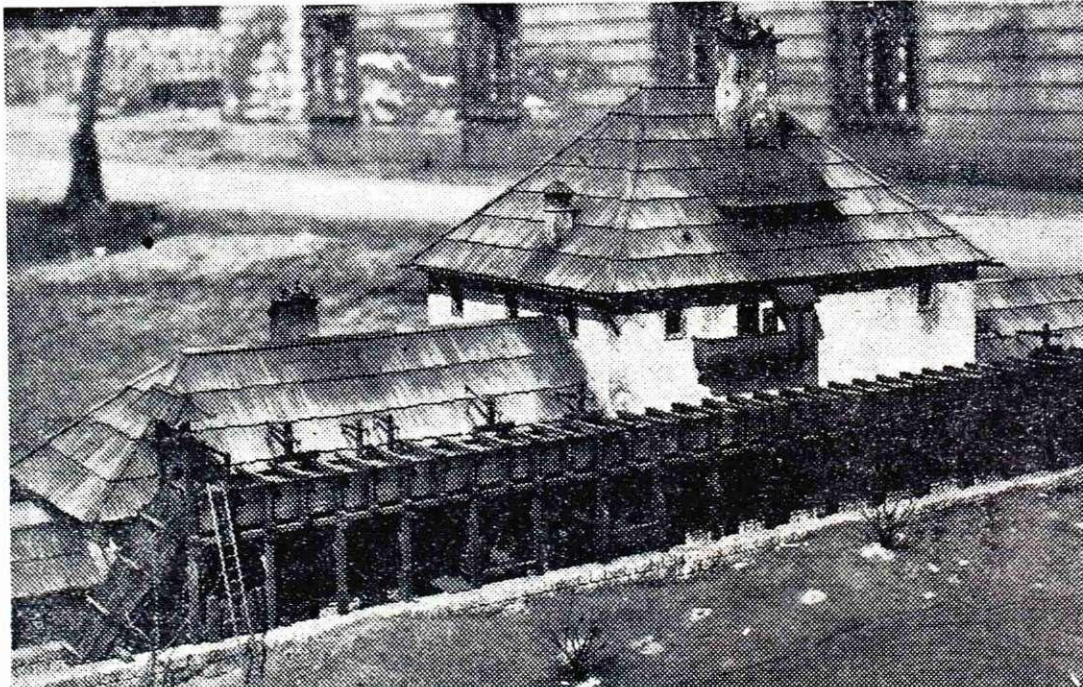
Maketa plavža na Javorniku iz leta 1796, ki jo je izdelal sodelavec tehniškega muzeja Marjan Dolinšek
