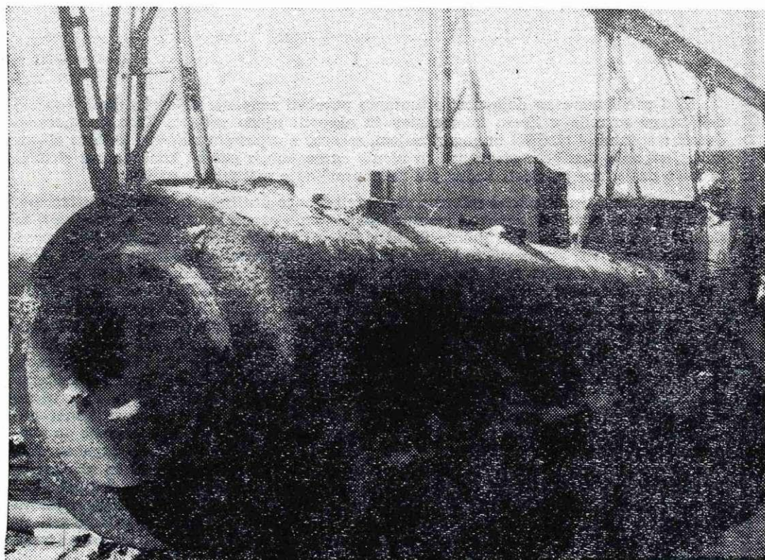
Naša jeklovilarna je izdelala dva odlitka za potrebe ladjedelnice 3. MAJ na Reki. Vsak tehta bruto 32 ton in je bil prevzet po prevzemnem organu Lloyd Registra. Prvega že obdelujejo na končne mere v Litostroju, drugi pa je bil odpravljen pred dnevi.
