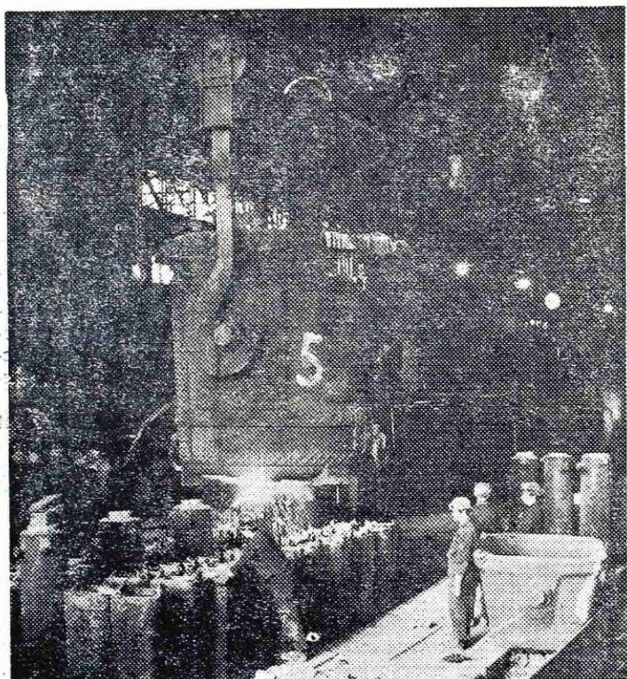
Vlivanje jekla v kokile (električna peč)
