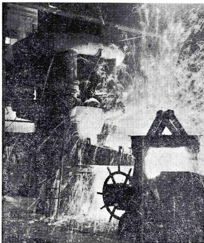
Prvi šarž iz nove kupolke v sivi livarni
