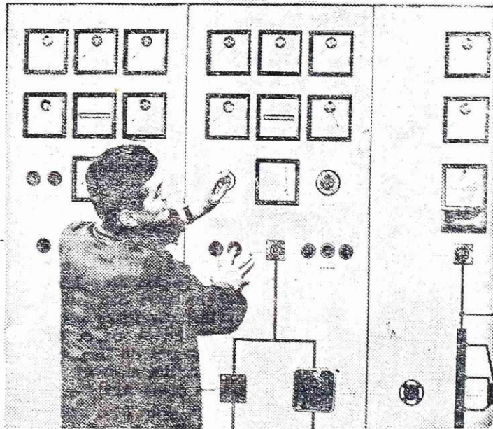
Preizkušnja elektromotorjev na preizkusni plošči
