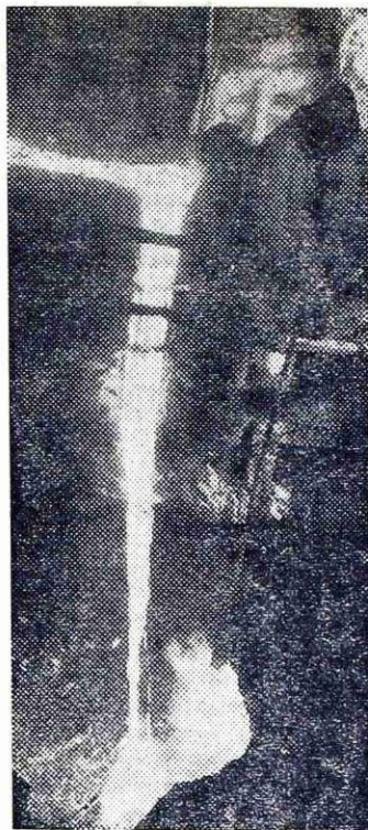
Kolektiv DE plavž si prizadeva, da bi bil grodelj kvalitetnejši in cenejši
