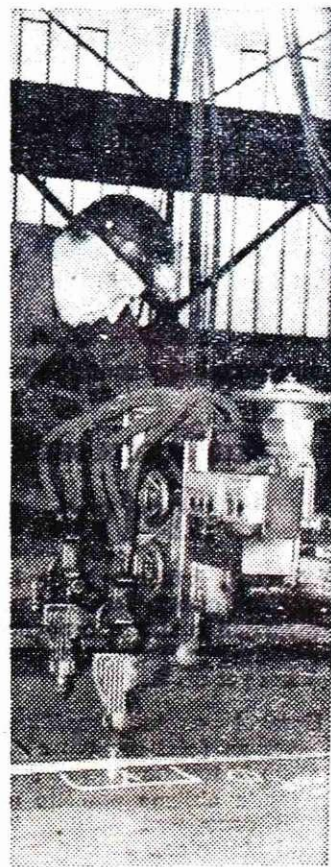
Avtogensko rezanje debele pločevine
