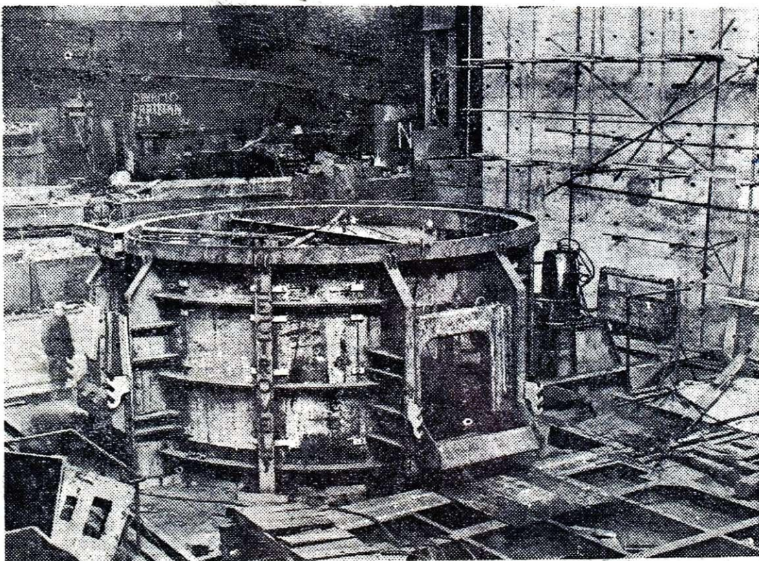
Izgradnja nove električne peči LECTROMELT
