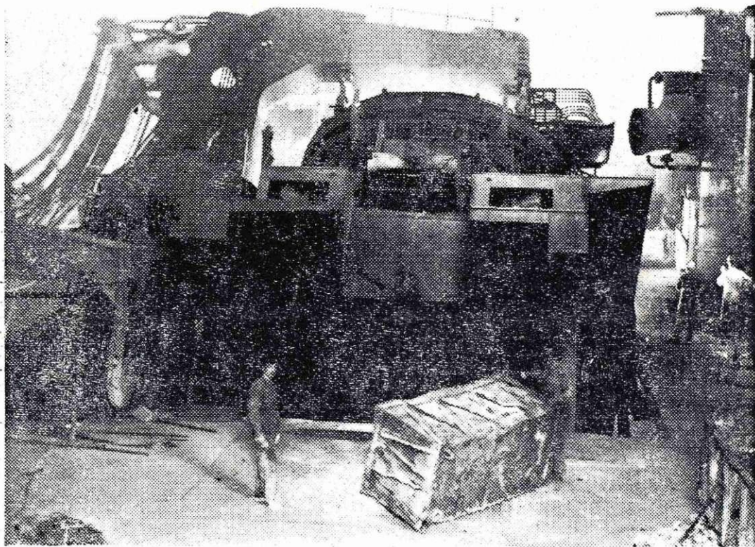
ASEA električna peč, se mora pri izlivu nagniti za 45 stopinj
