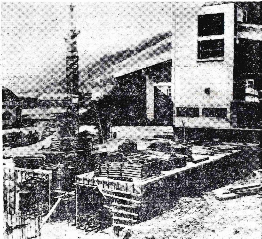
Na sliki objekt 04 - 100 m vsipnik, ki že obratuje in 136 m vsipnik v gradnji
