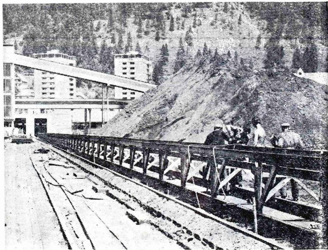
Vsa rekonstrukcijska dela v železarni so namenjena izboljšanju delovnih pogojev, pocenitvi proizvodnje in izboljšanju poslovne politike. — Na sliki dela na aglomeracijskih napravah
