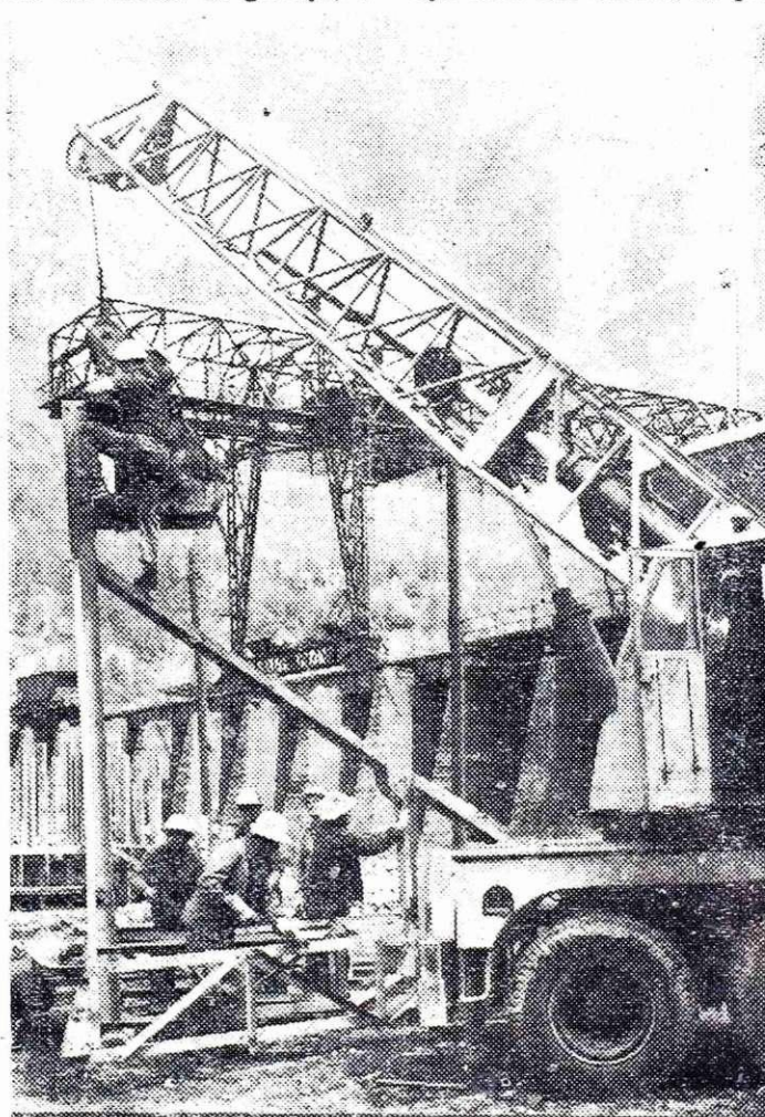
Montaža jeklene konstrukcije za objekt 22 v novih aglomeracijah
