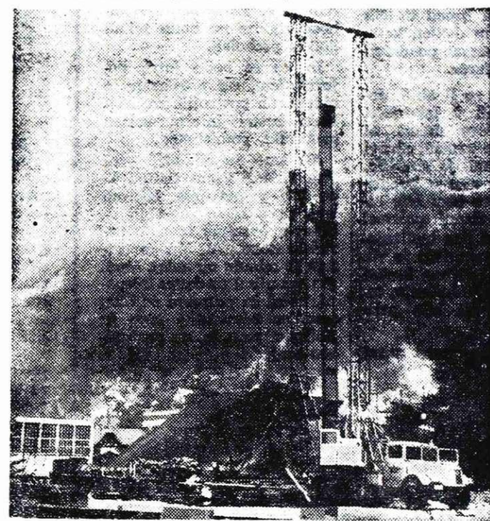
Prvi steber za novi objekt aglomeracije
