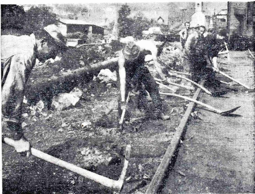
Gradnja novih aglomeracijskih naprav zahteva večkrat tudi prestavitve tirov
