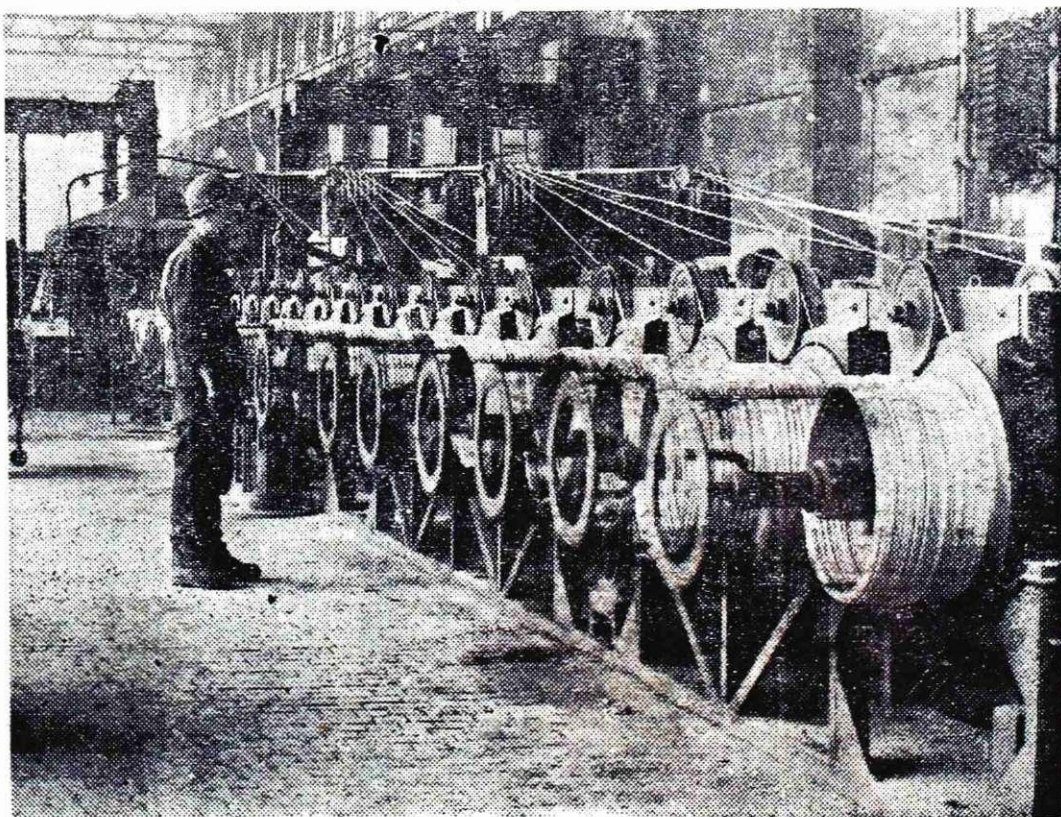
Pocinkovalnica žice v predelovalnih obratih — proga 3
