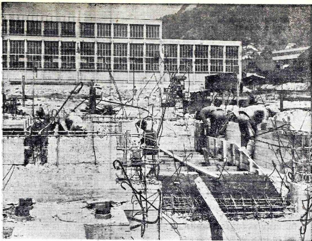
Nova aglomeracija — opažanje plošče 0,00, objekt 22
