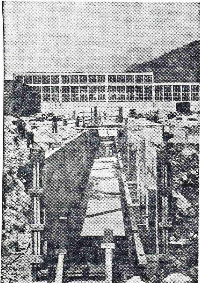
Novo aglomeracije — izkop temeljev in betoniranje kanalov
