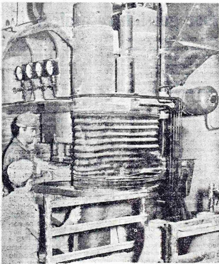
Nova 1000-tonska hidravlična stiskalnica
