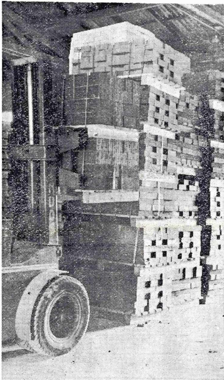
Končne izdelke paletizirajo in prevažajo z viličarji
