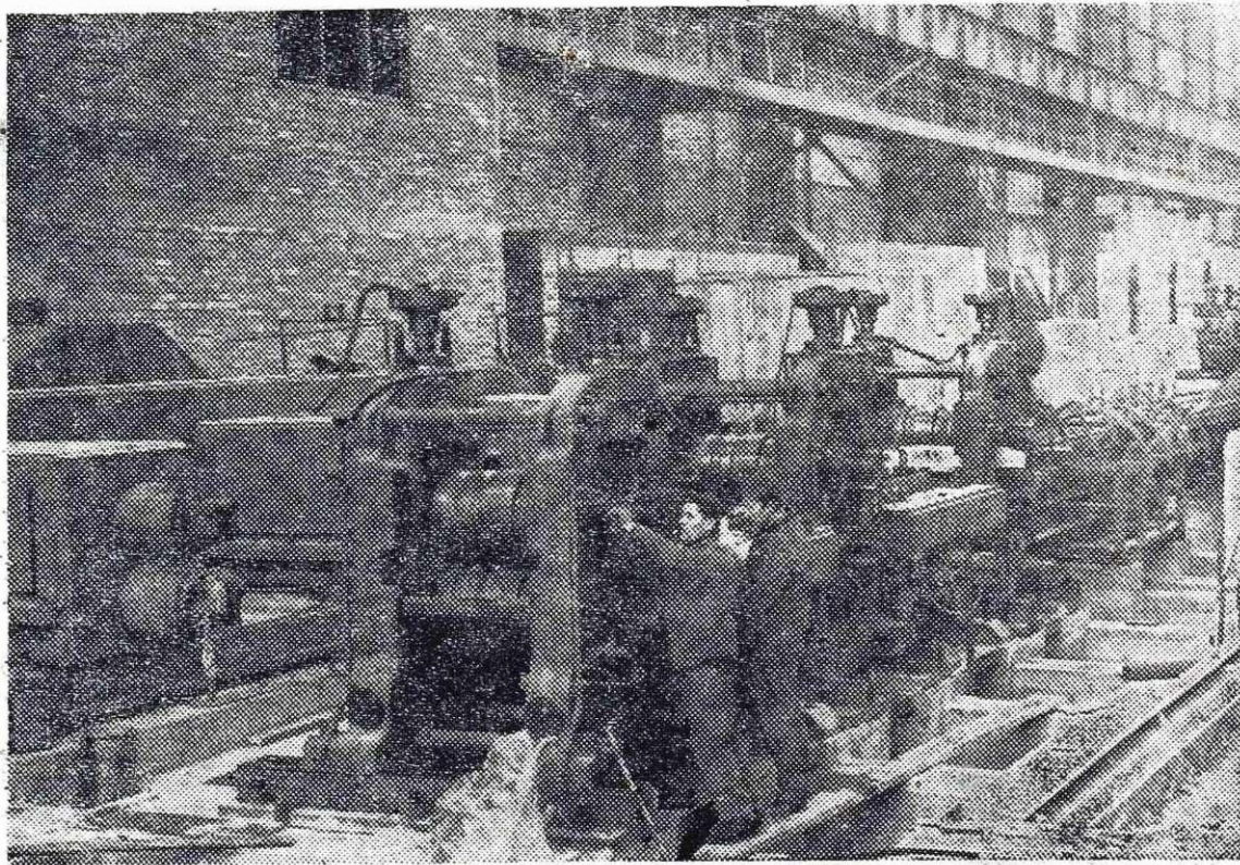
Montaža proge 450 v novi žični valjarni
