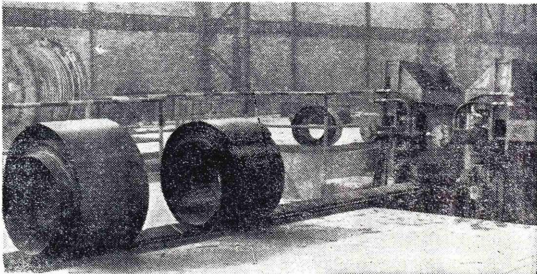
Verižni transporter za svitke v valjarni trakov na Beli
