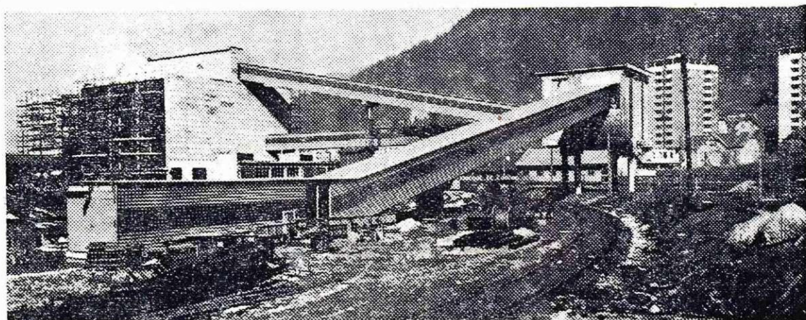
Obloga mostov za transportne trakove je lepa in ekonomična
